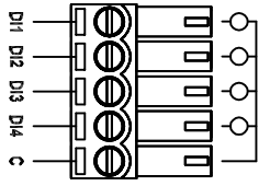
TB1
