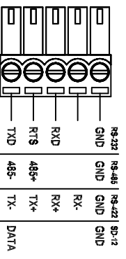
TB7 (COM1)
