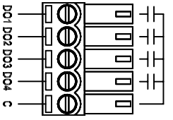
TB3
